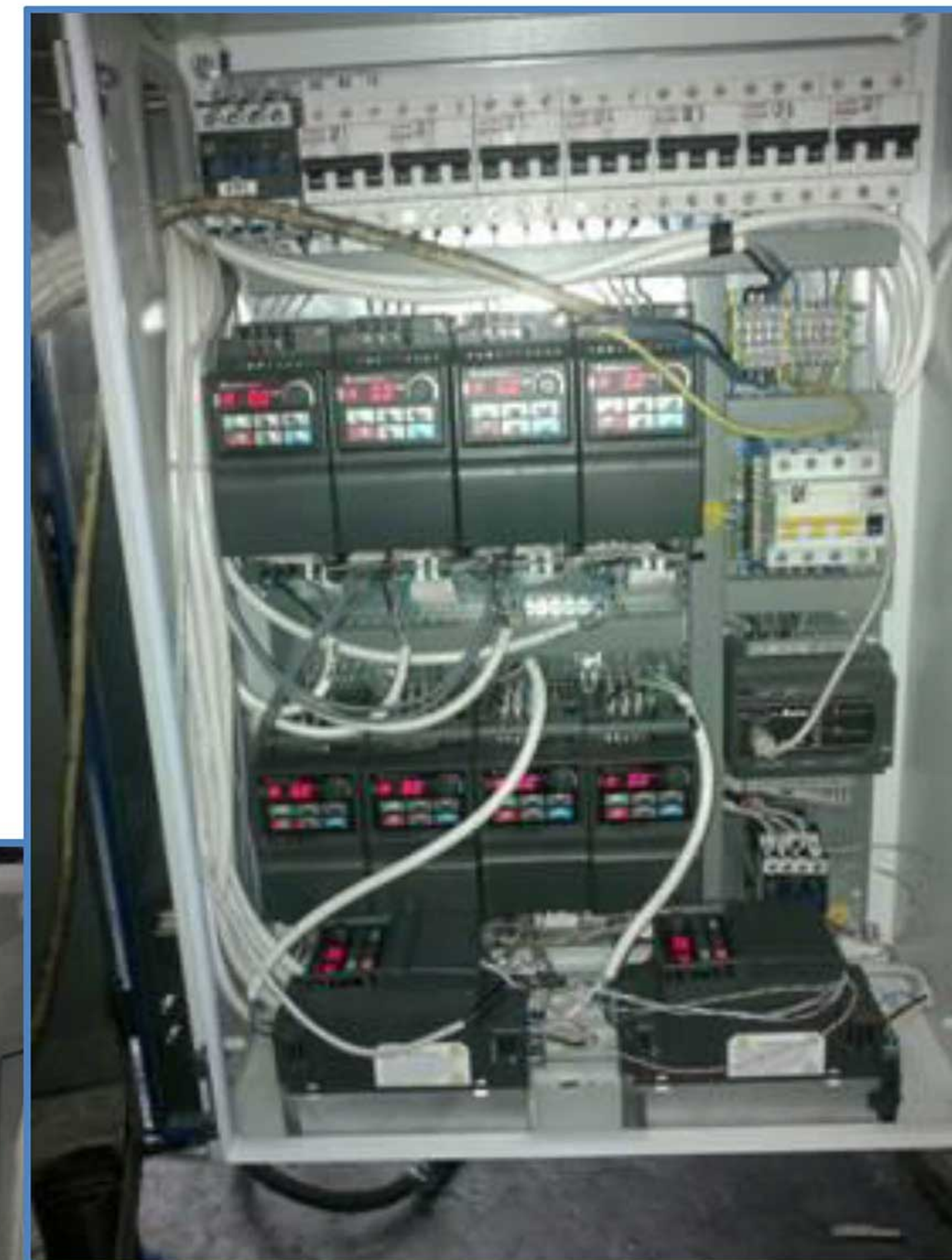
ПЧ VFD-EL и ПЛК DVP-ES2 в шкафу управления аппарата СД-800
